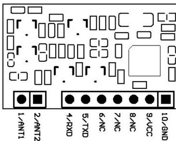
图 3-1 JY-LD6930 管脚图
